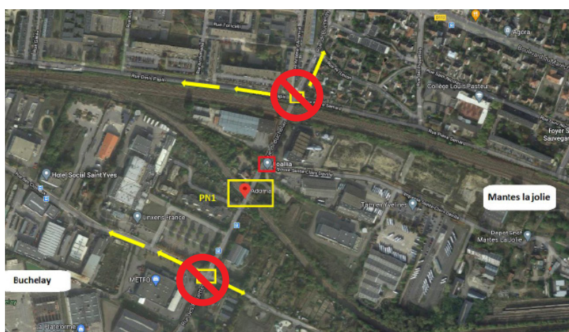
Nouvel ouvrage d'art rue de Buchelay - DRIC Projet Eole
